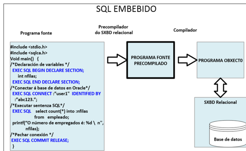
Exemplo do proceso de compilación dun programa con sentenzas SQL embebidas na linguaxe C
